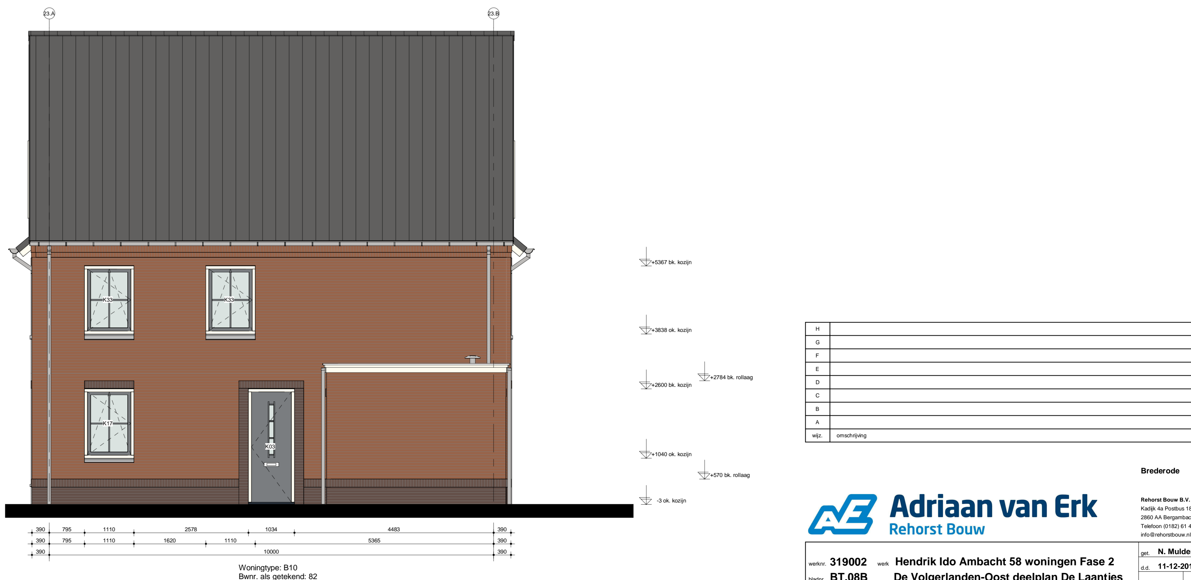
Rechtergevel blok 23
