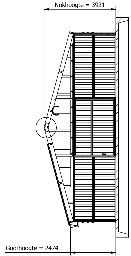
B-B ( 1 : 100 )
