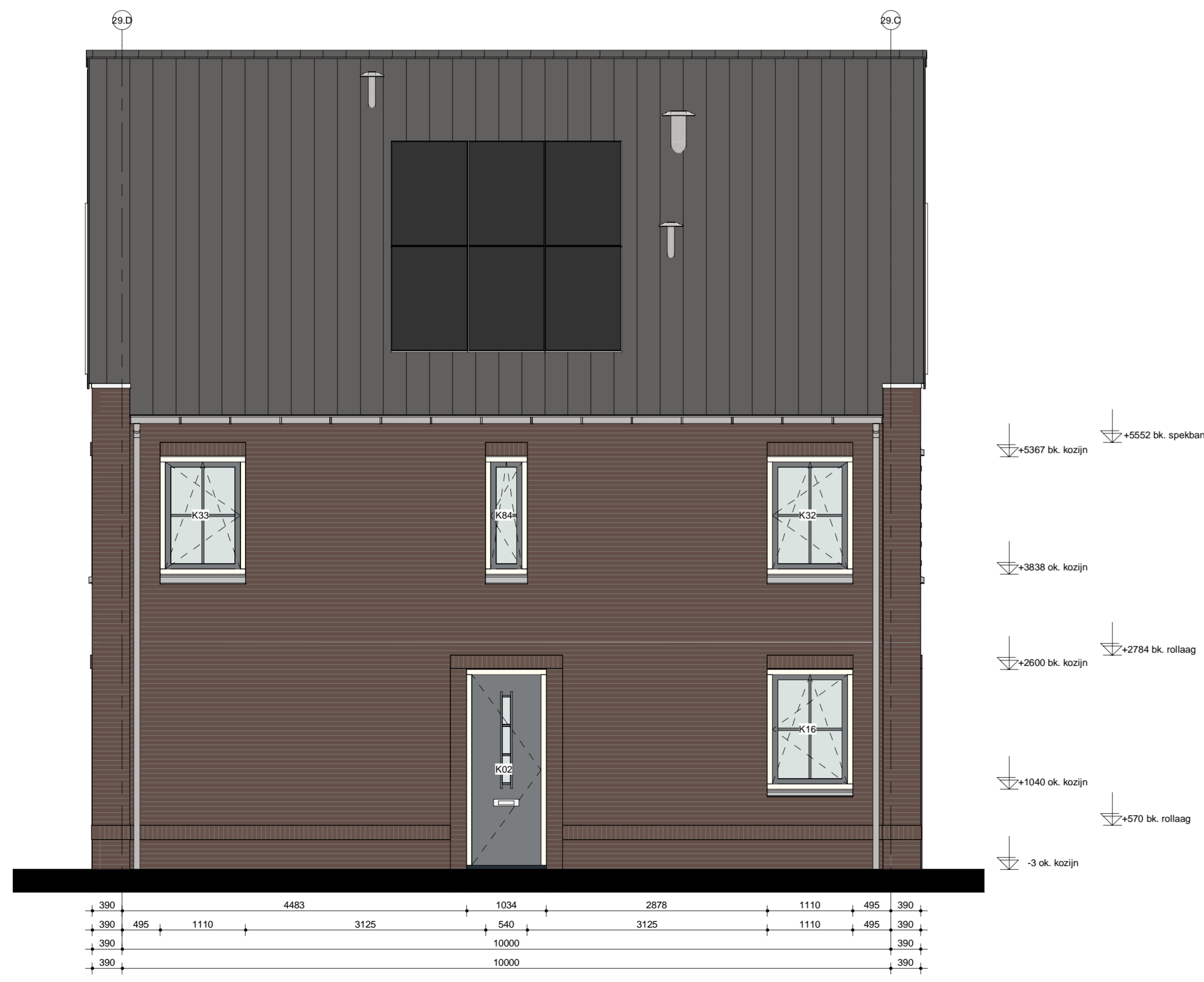
Linkergevel blok 29
