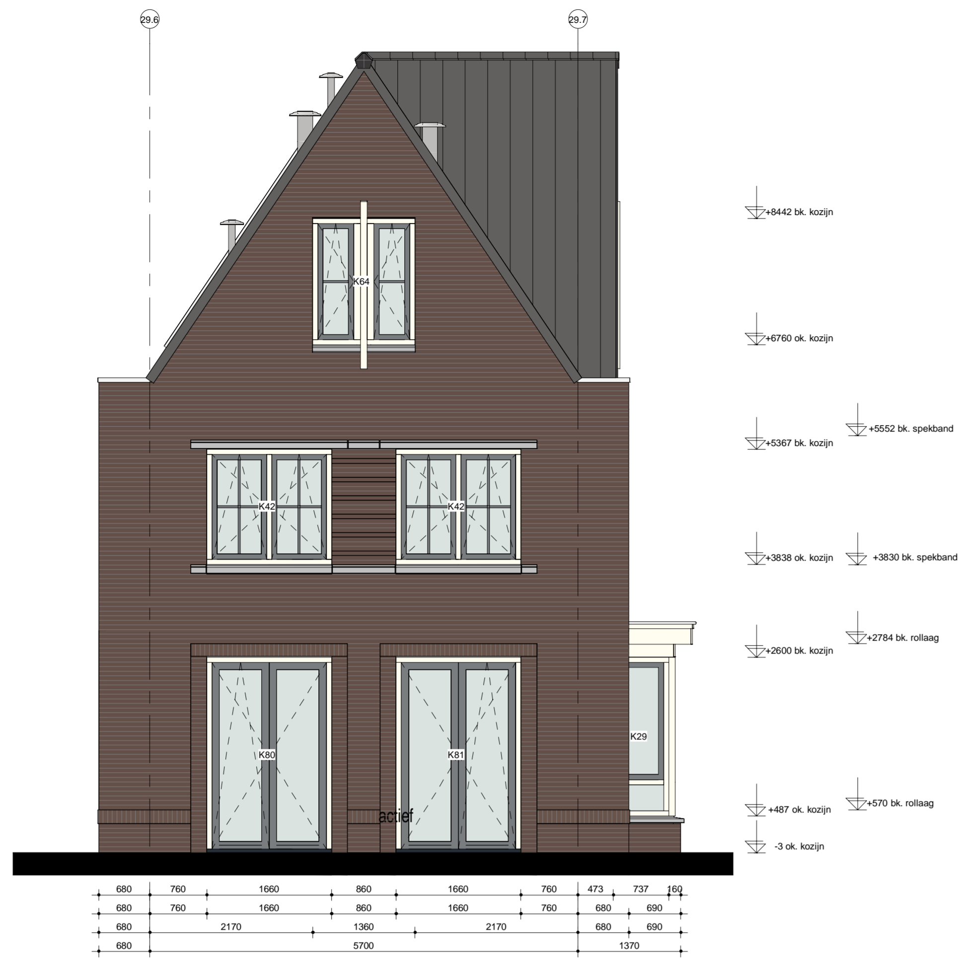
Voorgevel blok 29
