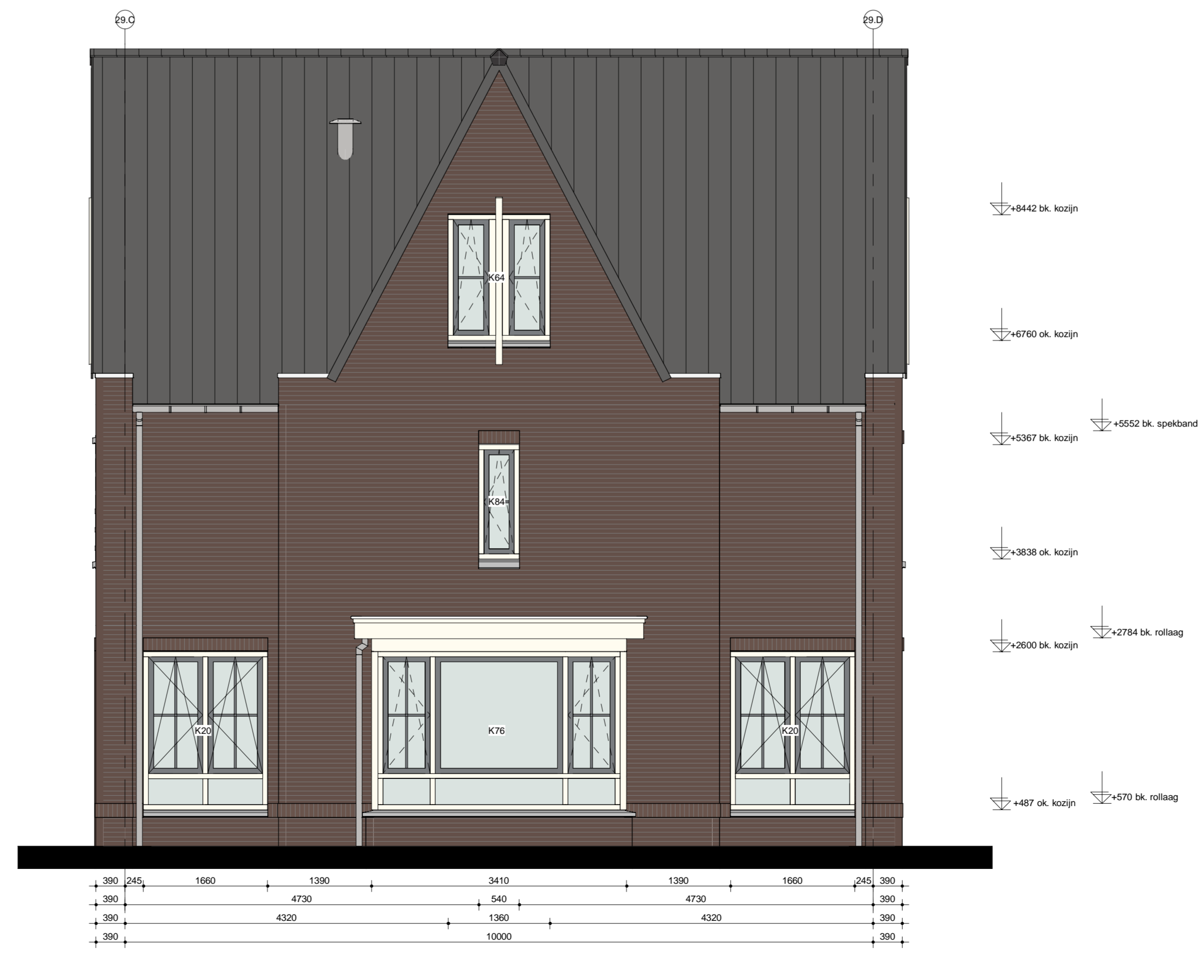
Rechtergevel blok 29
