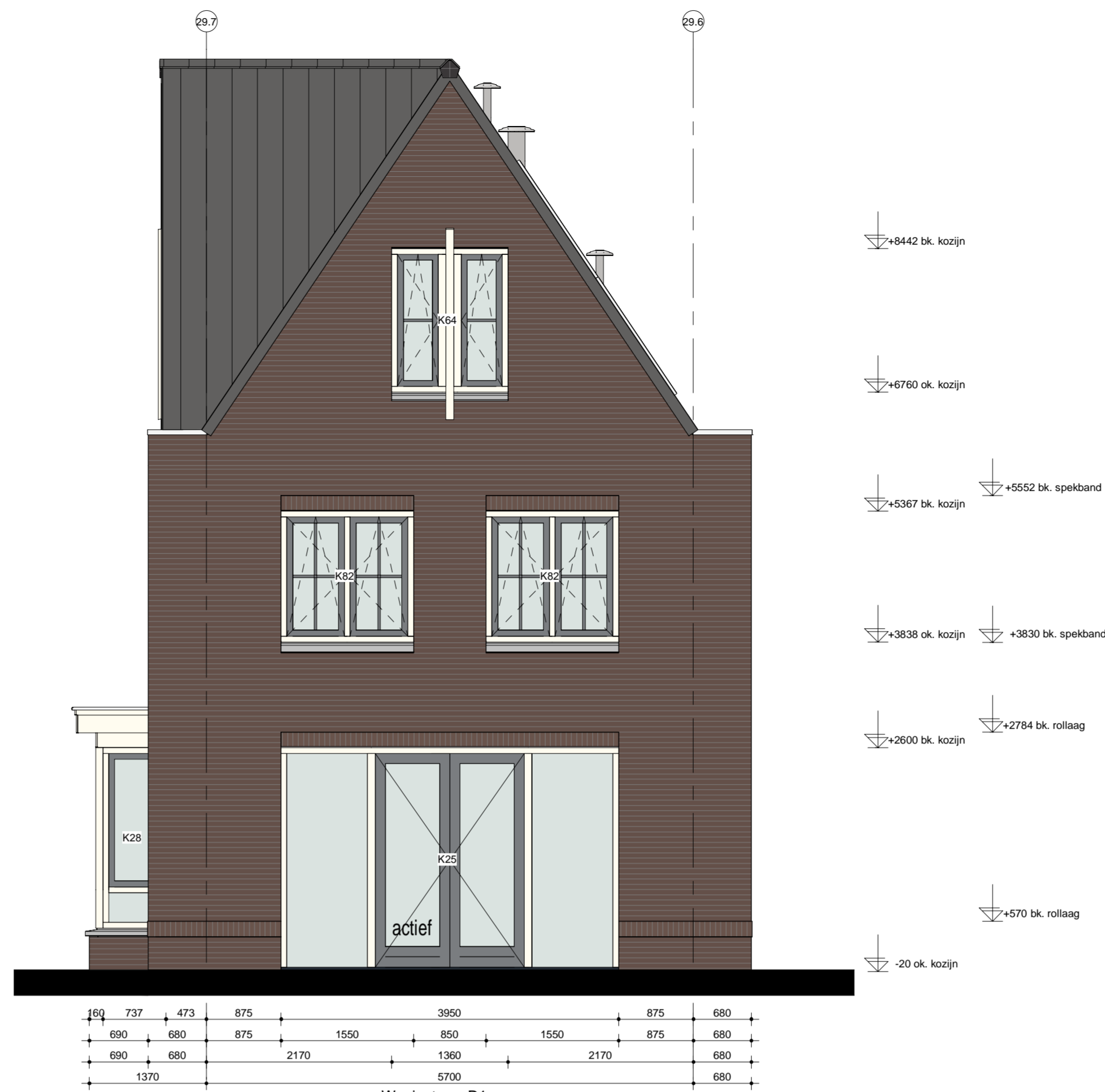
Achtergevel blok 29
