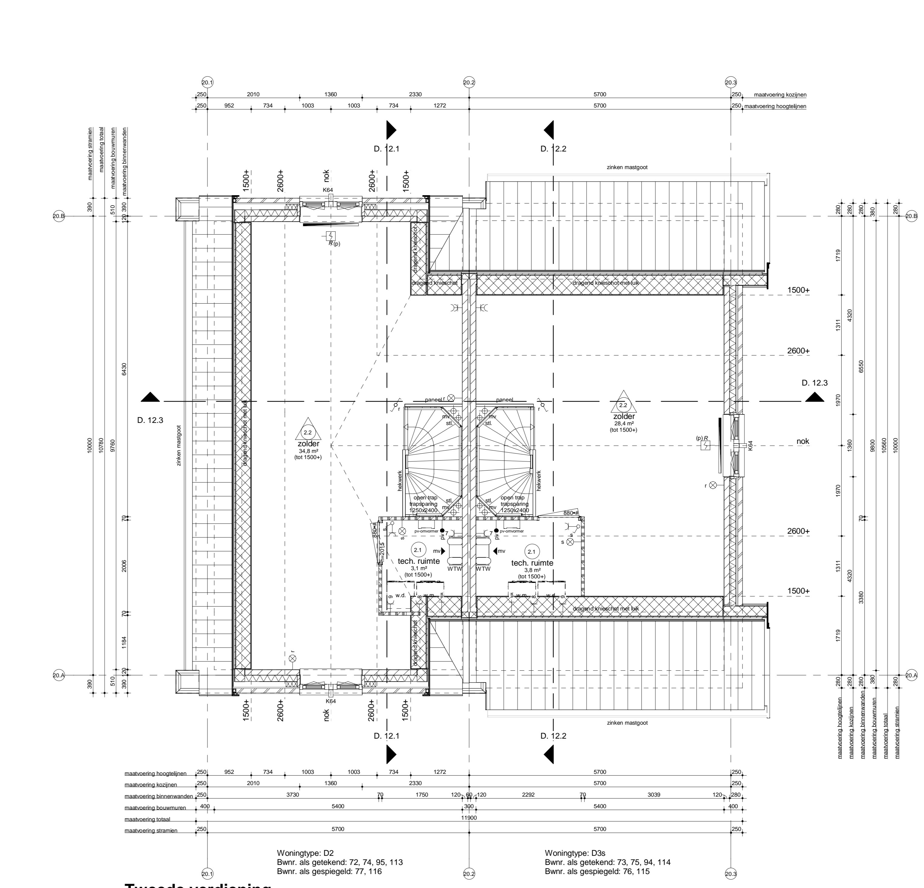
Tweede verdieping bk. vloer = 5900+vl blok 20, 29 & 35
