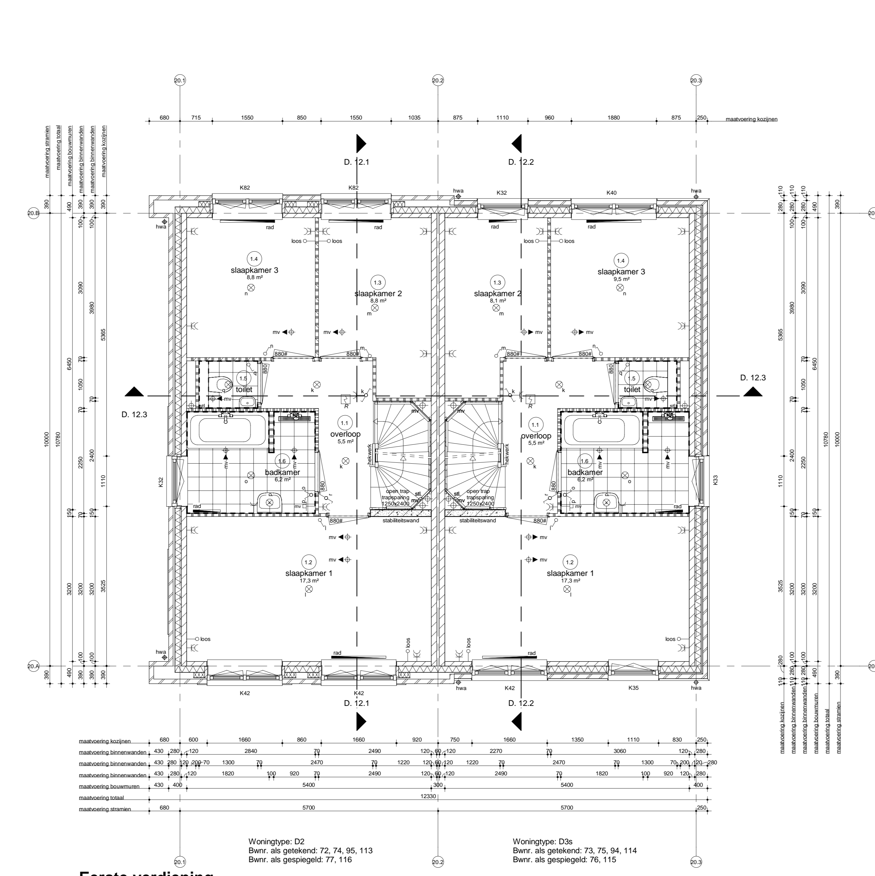
Eerste verdieping bk. vloer = 2950+vl blok 20, 29 & 35
