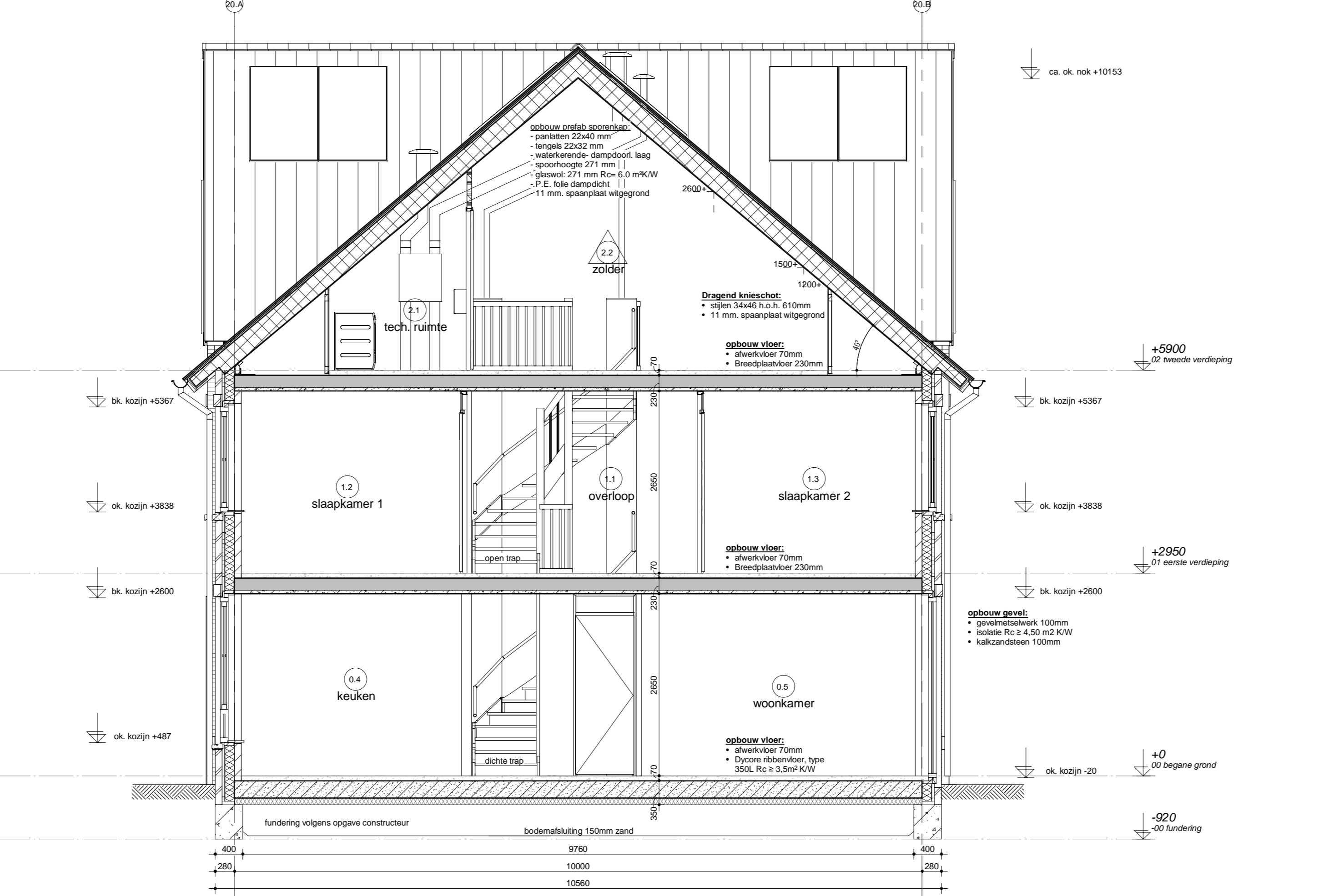
Doorsnede 12.2
