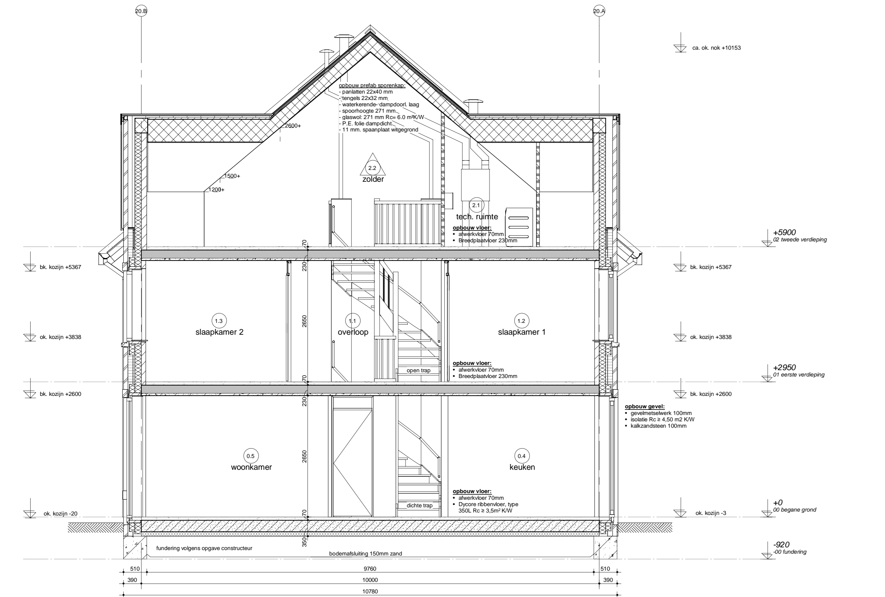
Doorsnede 12.1
