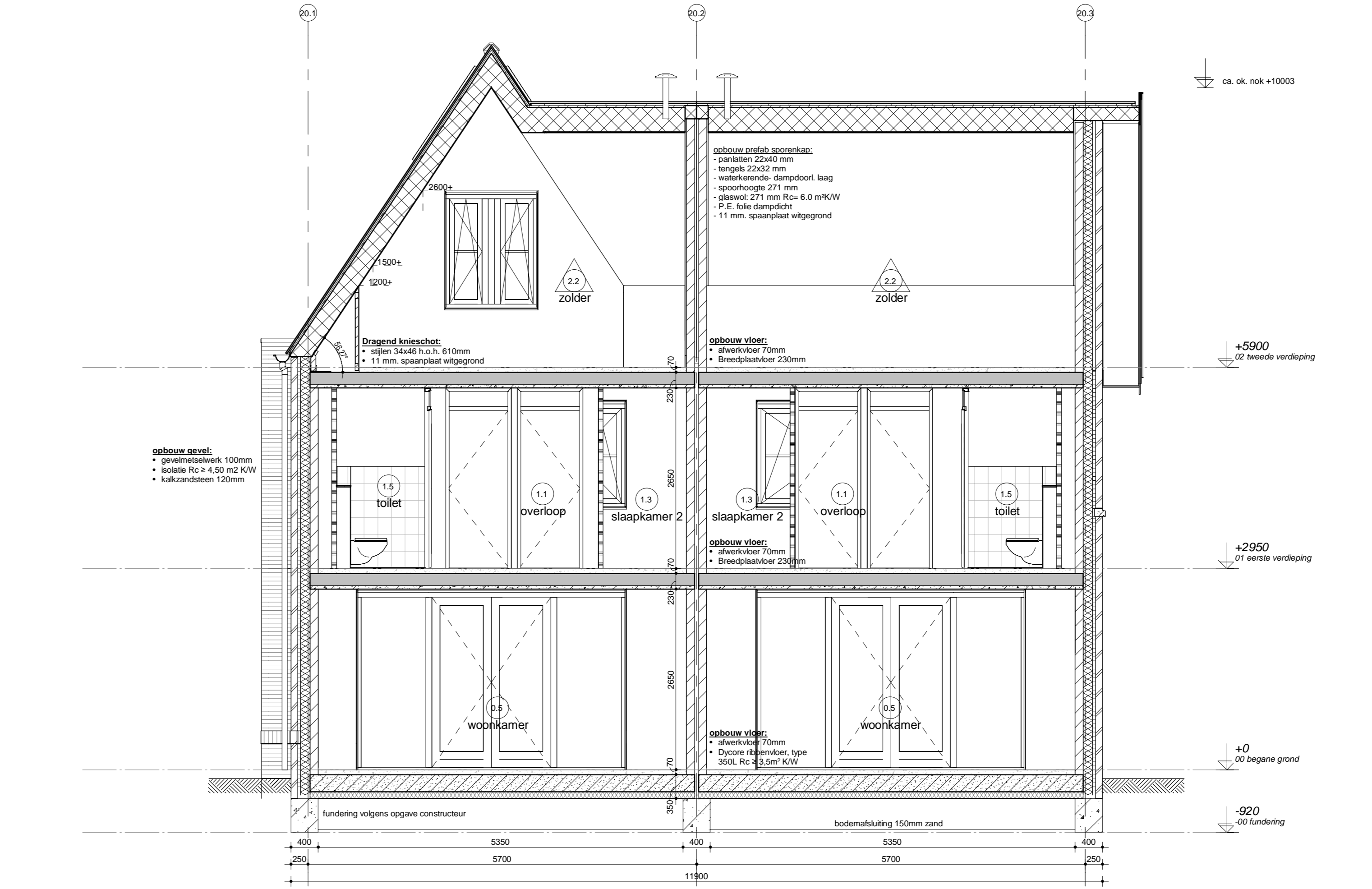
Doorsnede 12.3
